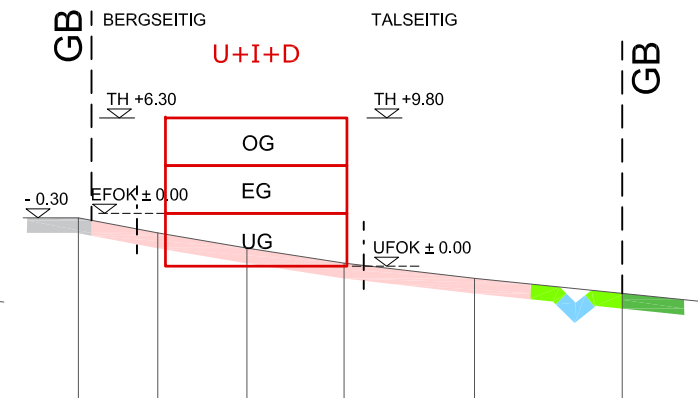
SCHEMASCHNITT FD
