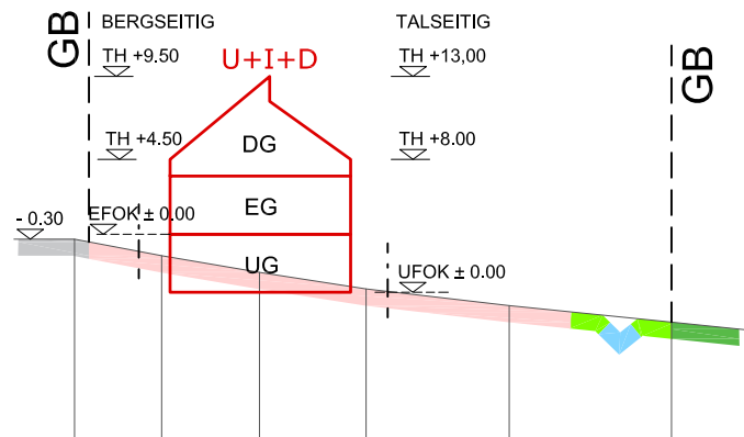
SCHEMASCHNITT PD
