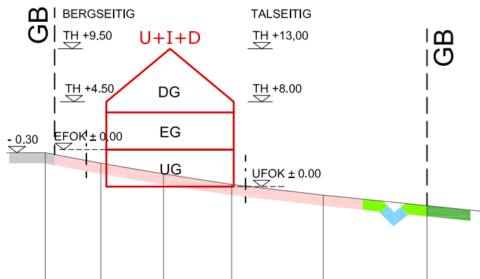
SCHEMASCHNITT SD
